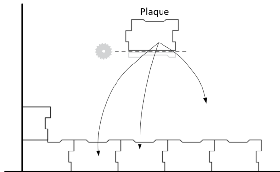
Schéma de découpe et démarrage de pose N°2
