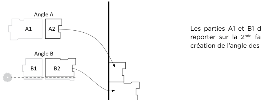
Schéma de découpe et démarrage de pose N°1
